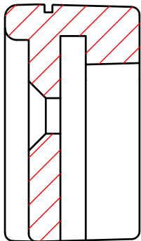
A-A ( 1.5:1 )
