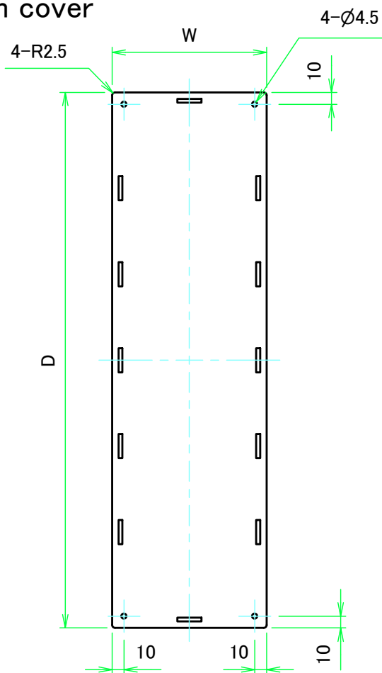
上カバー表面 / Top cover Frontside
