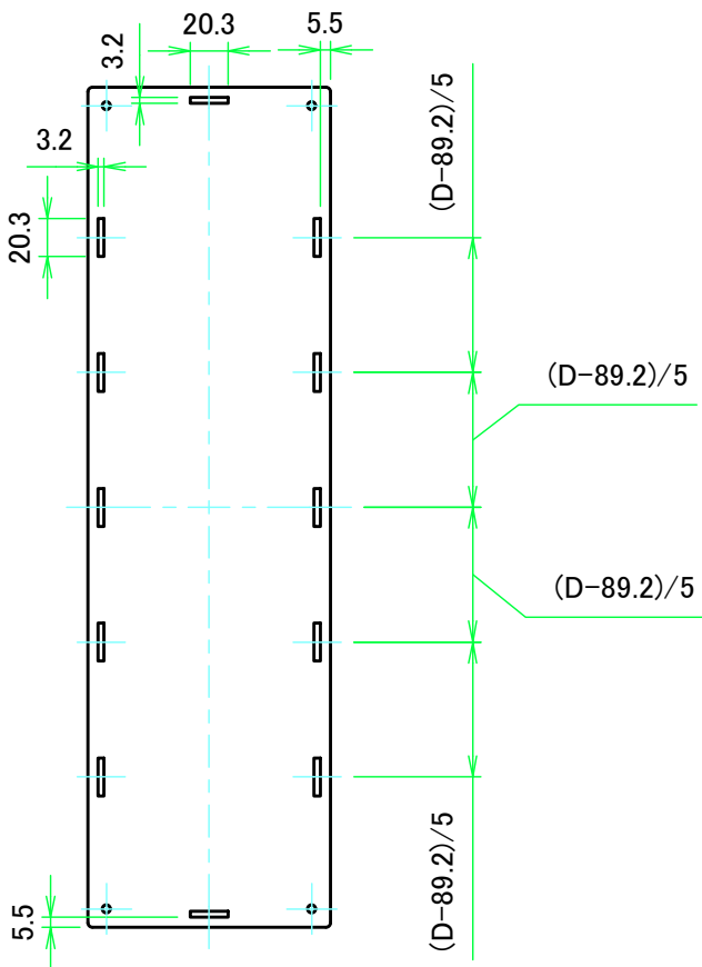
上カバー裏面 / Top cover Backside
